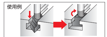
T溝上部からのセッティングが可能
