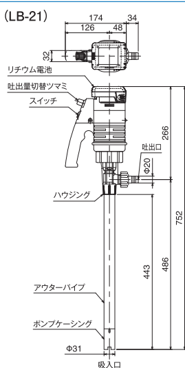
■ 寸法図 (LB-21)
