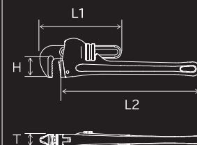
寸法図
