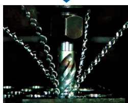
A-SFT シリーズ スパイラルタップで加工した場合の切りくず (オレンジブック 1-363 掲載品)
