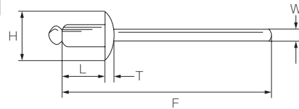
寸法図
