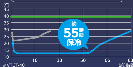
真空断熱クーラーボックスのボックス内温度の比較
