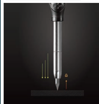
パワーロック機構により 2kgまでの荷重に耐えられる 芯保持力
