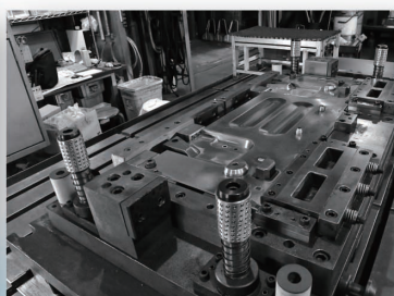
金型成形機
