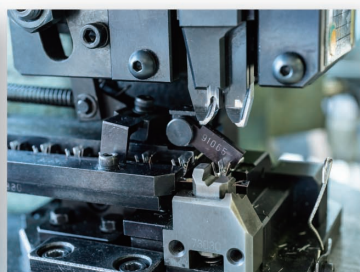
プレス機
