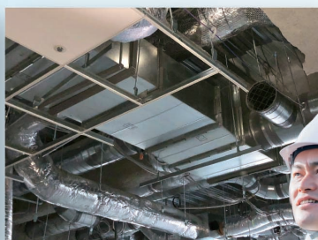
ダクト
